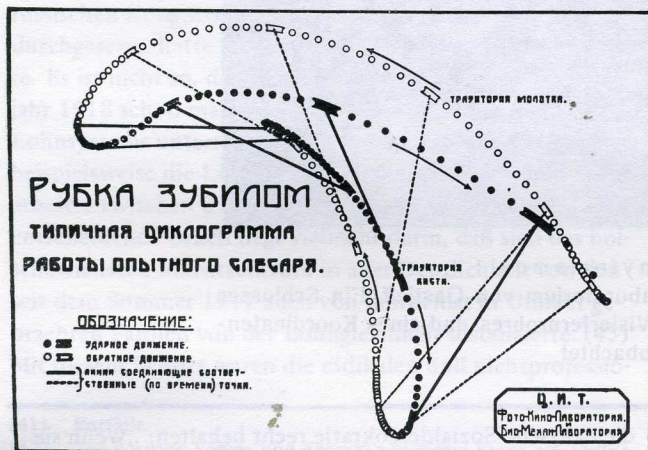
Zeitbahndiagramm über die Bewegung eines Hammers während des Meißelns (Institut Gastjeff)
